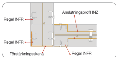
Bild 3. Hörn alternativ 1
