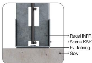
Bild 1. Golv-/takanslutning
