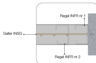
Bild 2. Väggstart
