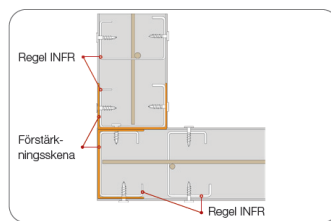
Bild 4. Hörn alternativ 2
