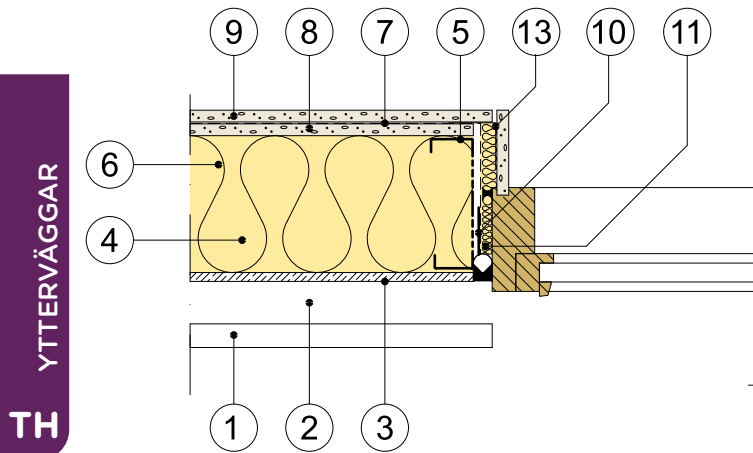
A Horizontalsnitt
