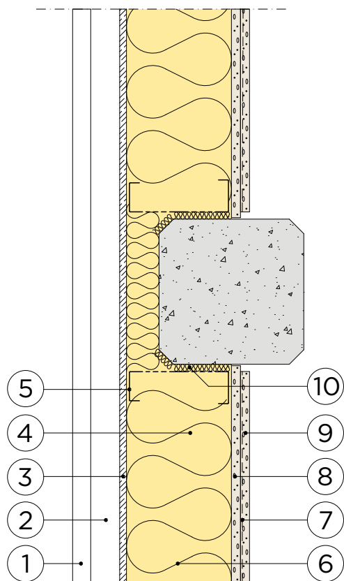
B Horizontalsnitt
