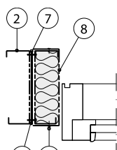
D Horizontalsnitt, 3-3
