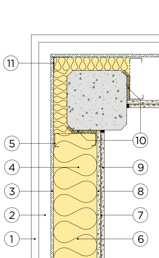
A Horizontalsnitt
