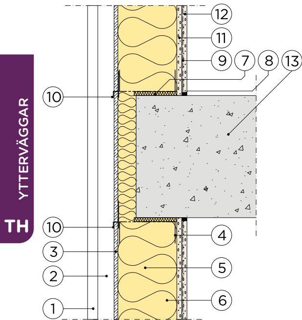
A Vertikalsnitt
