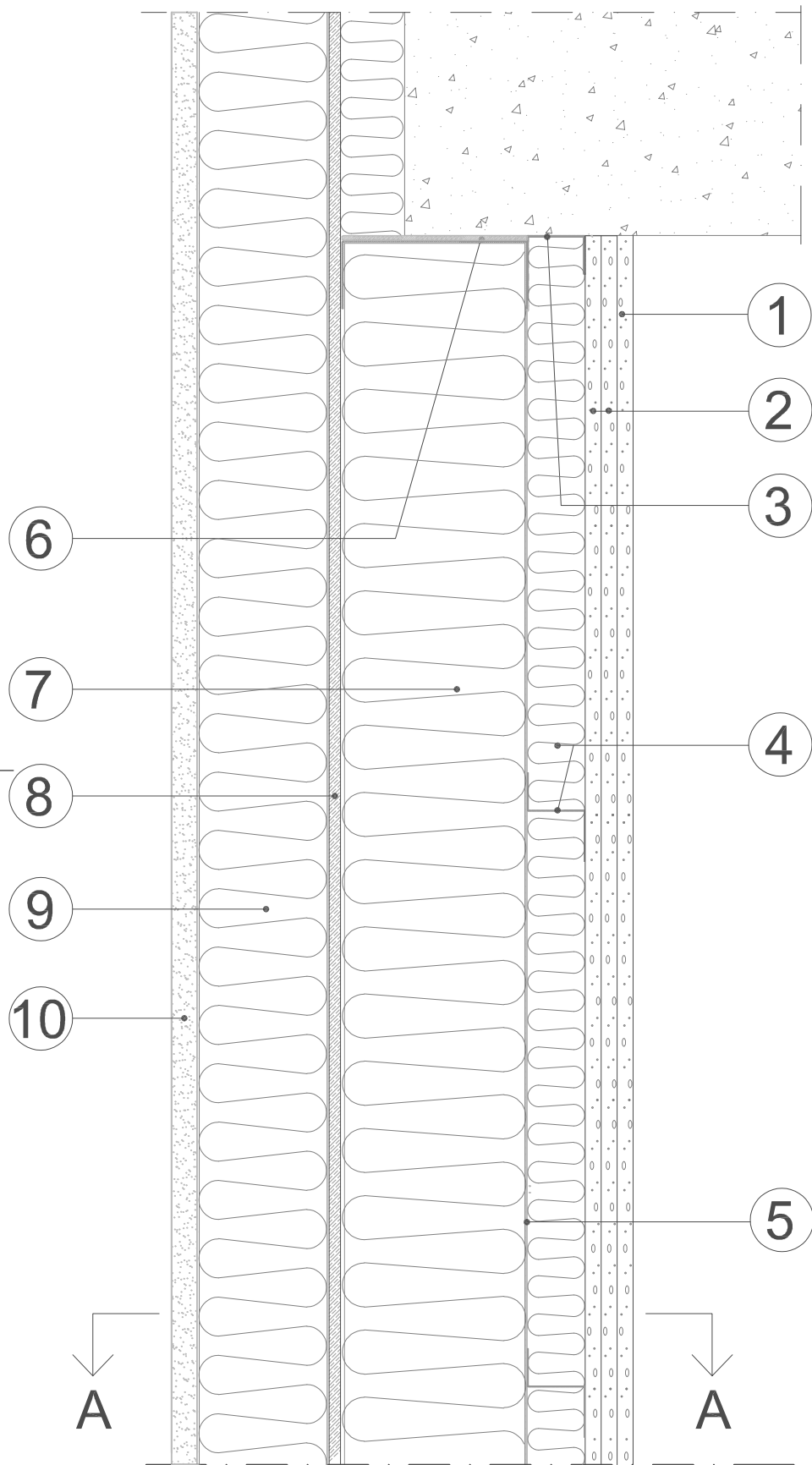
Vertikalsektion, 1:5
