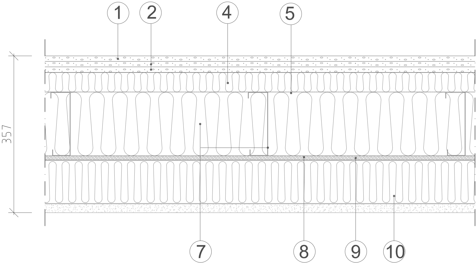
Horisontalsektion A - A, 1:5
